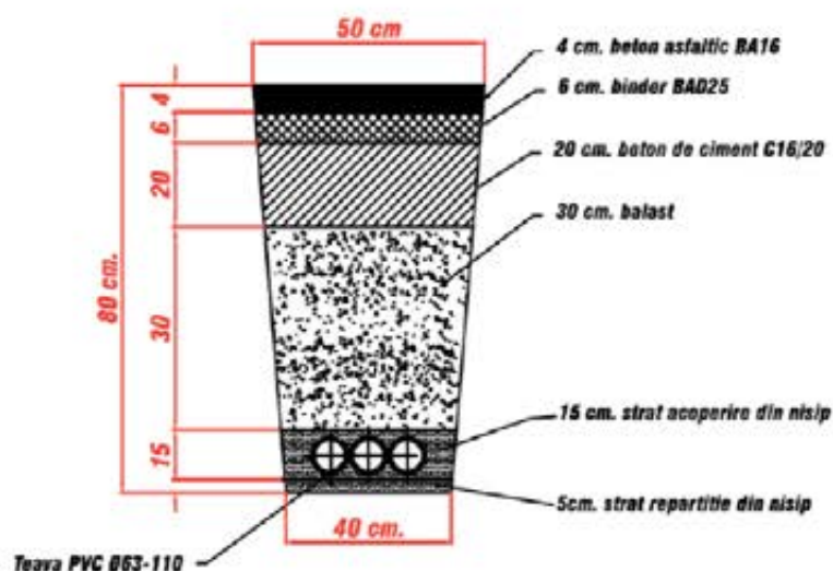
Figura 15 – Detaliu de instalare a infrastructurii de electroalimentare și date (exemplu)
